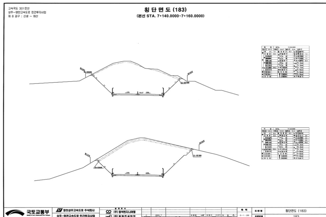
【그림 51.1.5】 표준횡단면도
